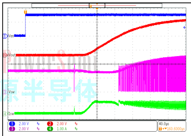
V_{IN}=3V , R_{LOAD}=20\Omega
