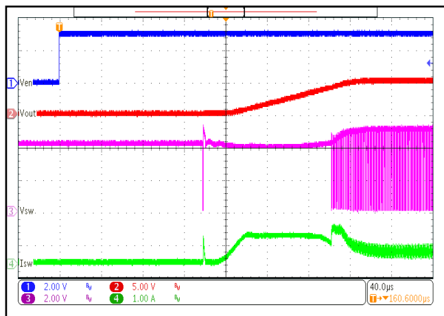
V_{IN}=4.2V , R_{LOAD}=20\Omega
