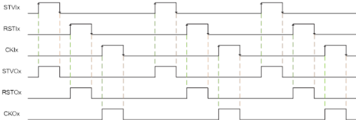
Figure5. TCON Mode
