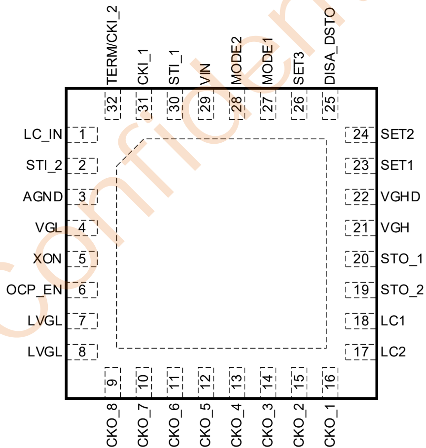
LPQ6274QVF QFN4X4-32
