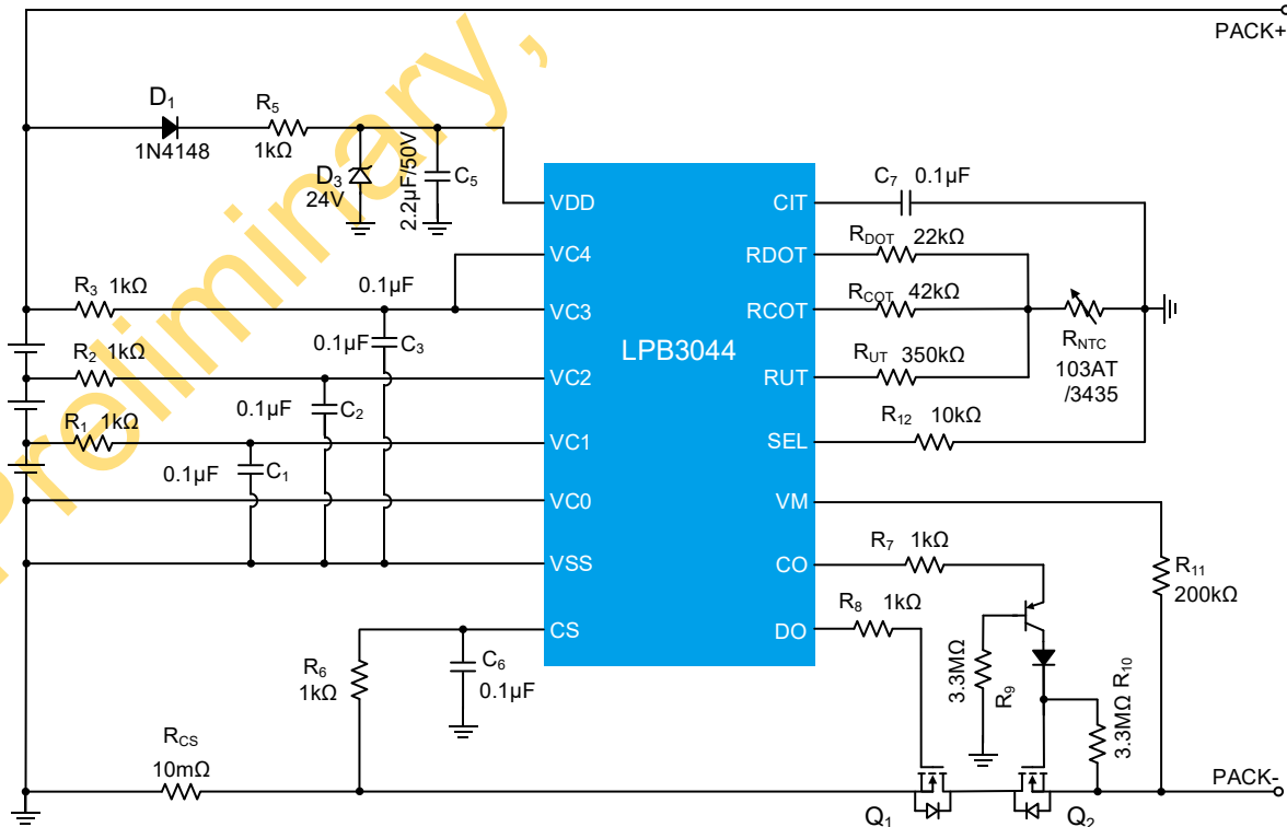
3串不带外部均衡功能同口应用电路图
