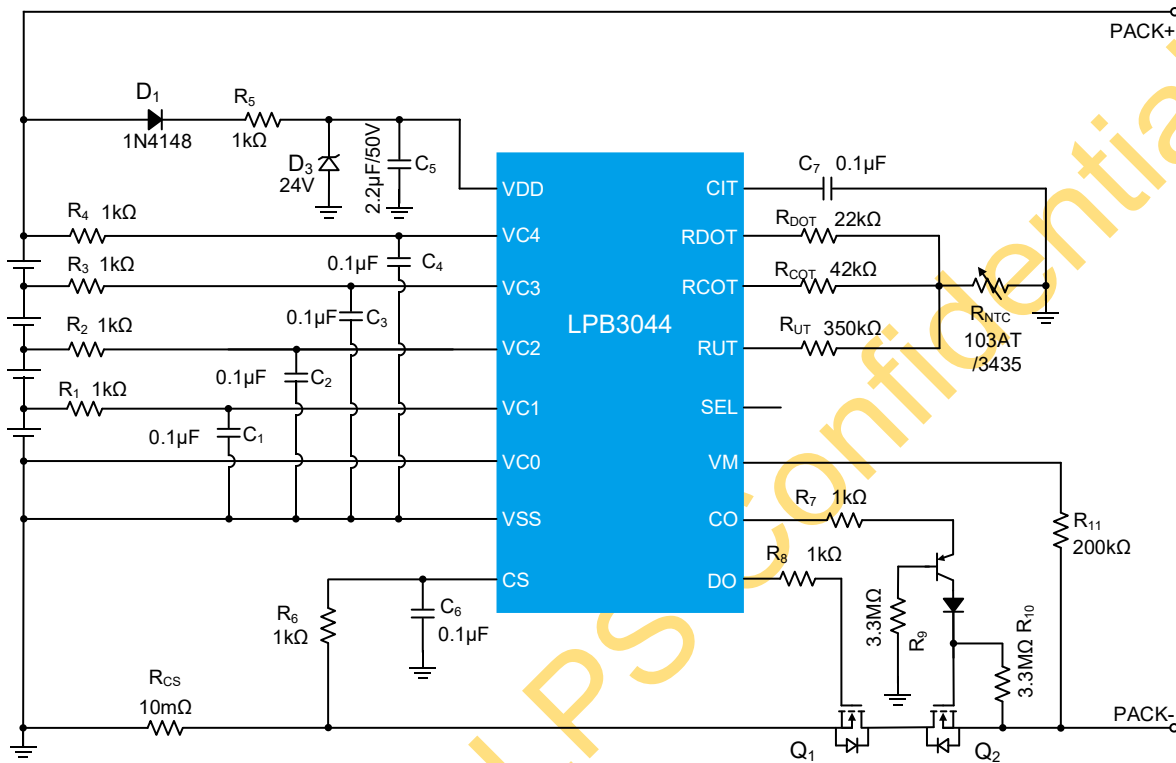
4串不带外部均衡功能同口应用电路图
